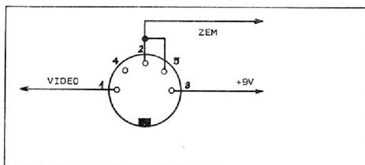
Obr.2 Zapojení konektoru pro TV
