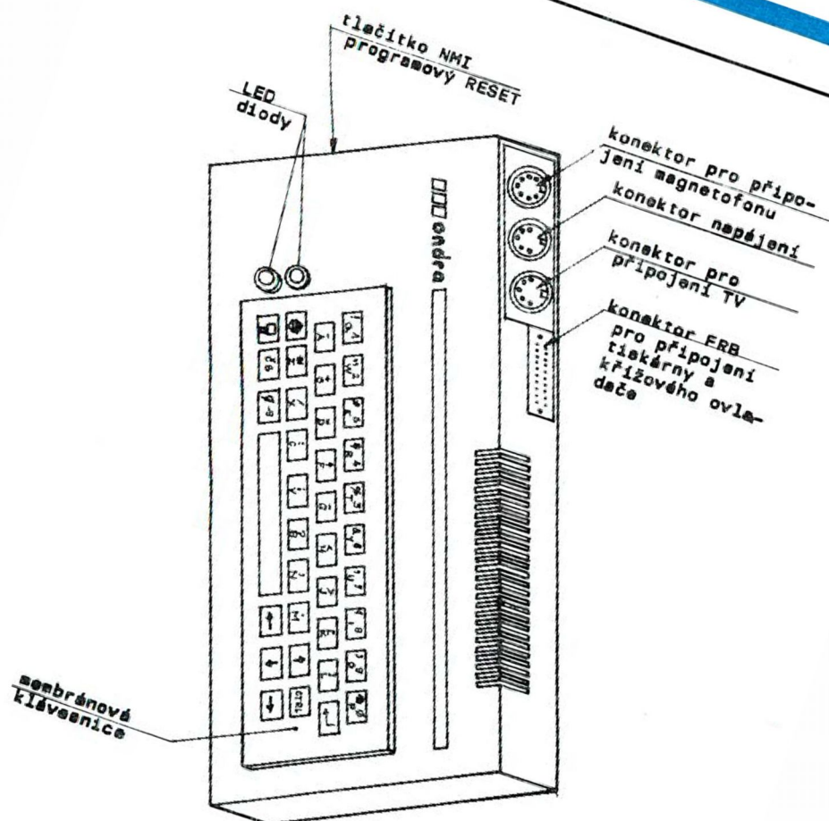
Obr. 5 Ovládací prvky a konektory mikropočítače ONdra
