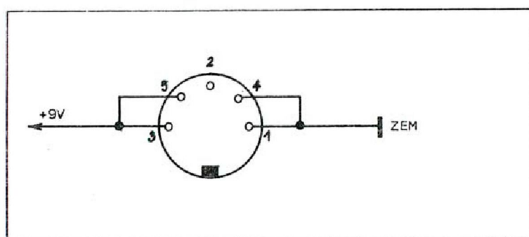
Obr. 3 Zapojení konektoru napájení
