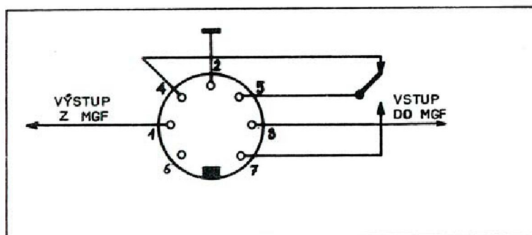
Obr. 1 Zapojení konektoru pro mgf
