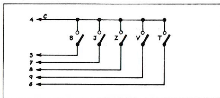
Obr. 4 Připojení křížového ovladače
